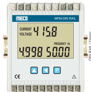
MFM-DIN RAIL
